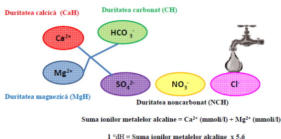
Figura 2. Componentele care dau duritatea apei (Eßlinger, 2009)
